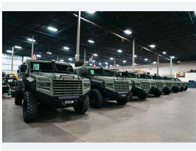
APC MRAP – otra vista de la fila de vehículos
